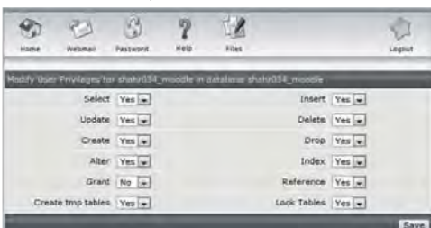
شکل ۲.۱۰. اختصاص دسترسی‌های لازم به کاربر پایگاه داده
